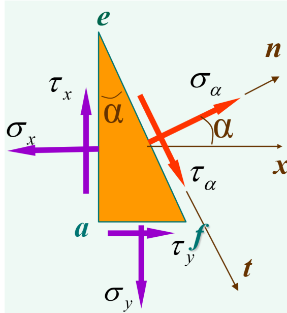
图 15: 斜截面上应力
